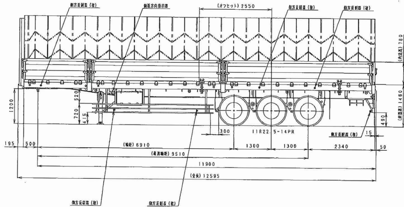
東急TF36H2C3型 セミトレーラ全体図
