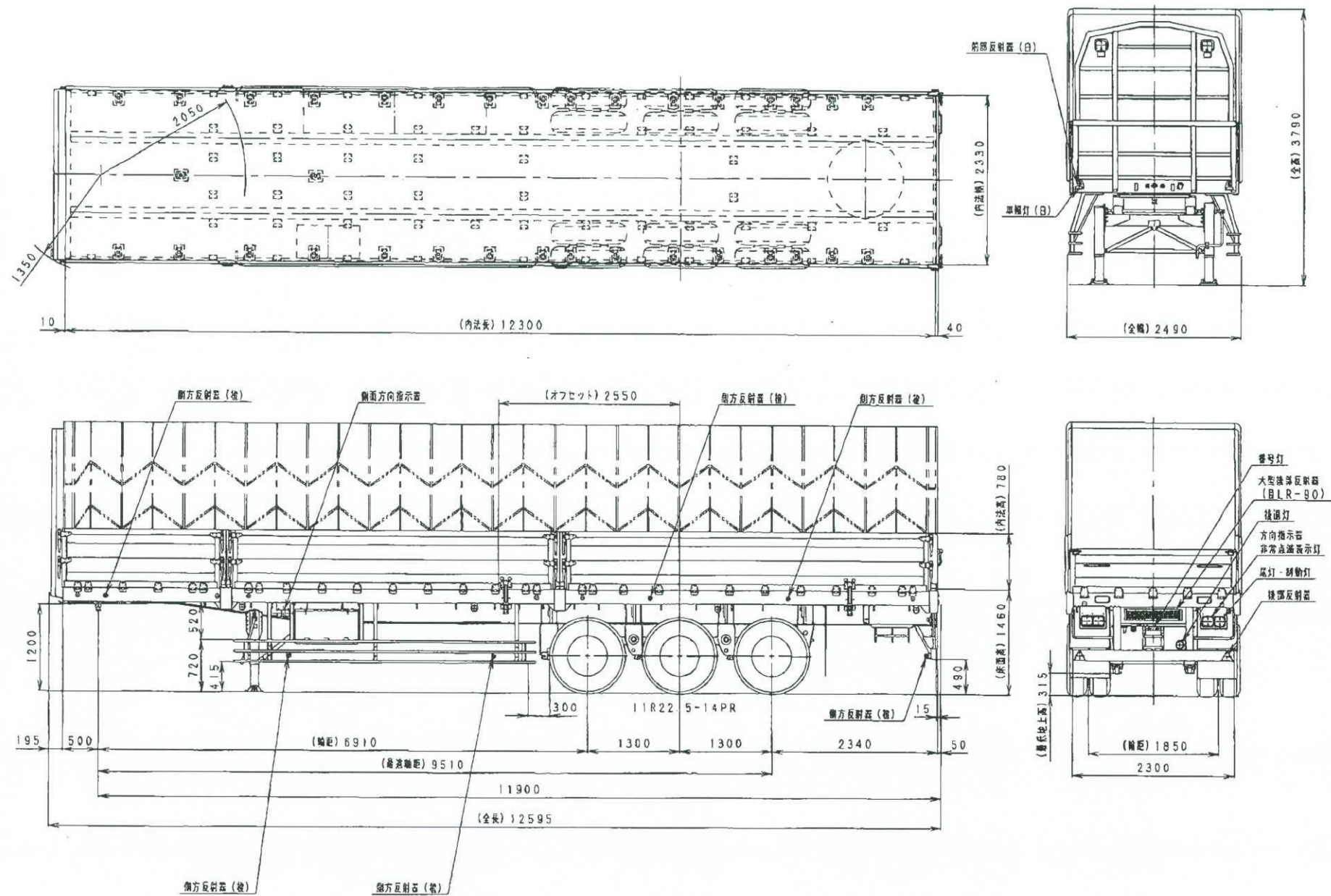
東急TF36H2C3型 セミトレーラ全体図
