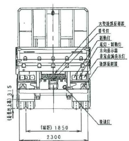
東急TF31H8C2S型 セミトレーラ外観四面図
