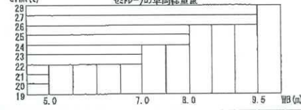
セミトレーラの車両総重量
